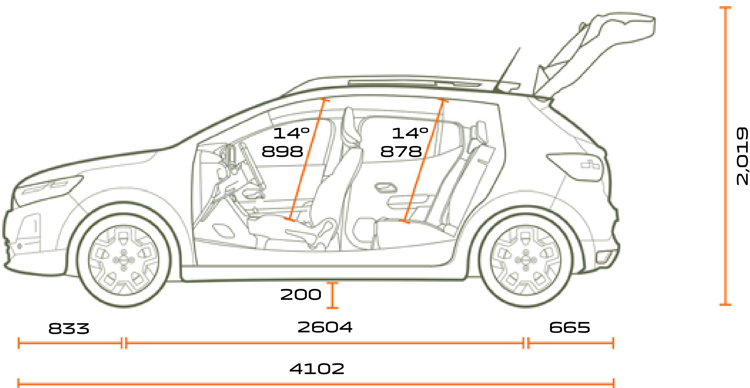
VISTA LATERALE
