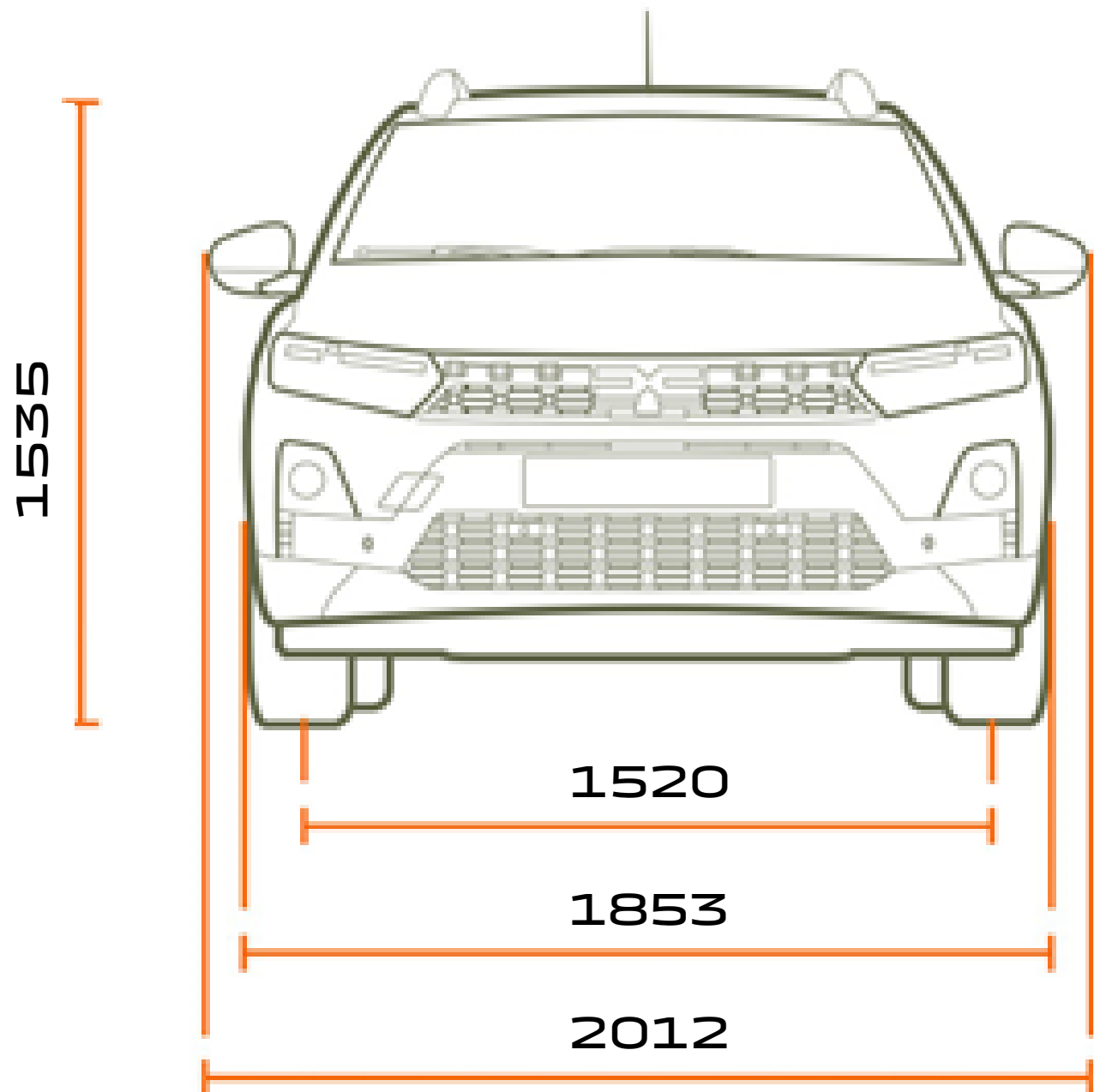
VISTA FRONTALE
