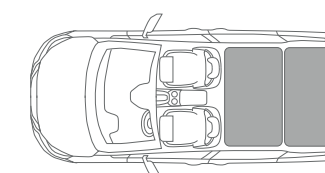
volume di carico: 3,9 m 3 lunghezza di carico: 1.806 mm x2 Europallet
